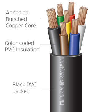
RV Cable
